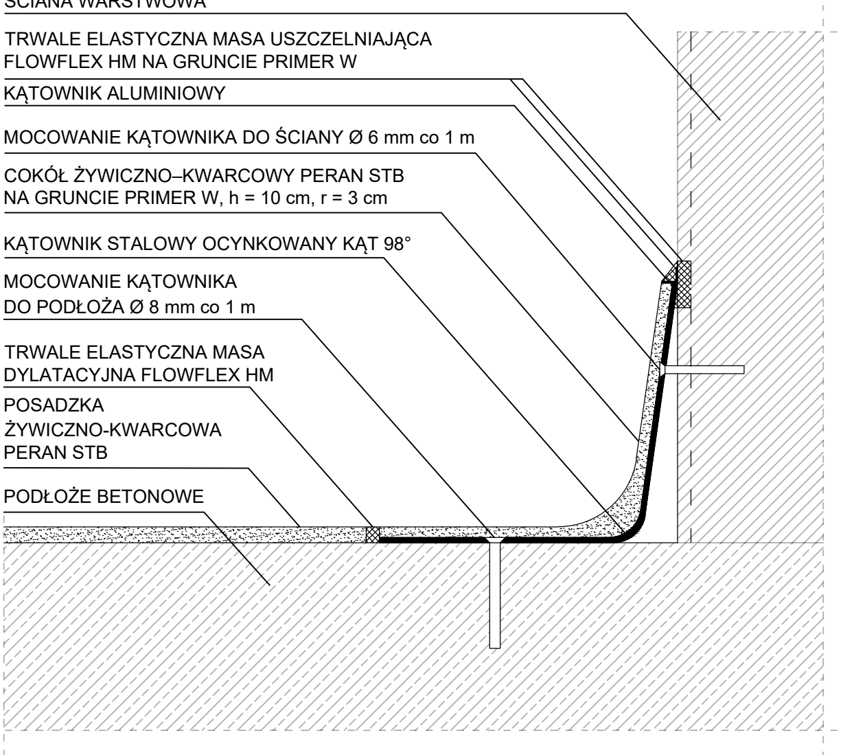
Rysunek schematyczny
